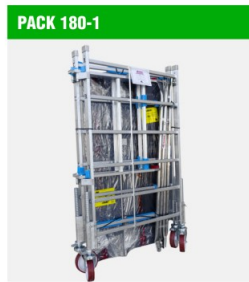
Módulo base: - Laterales, travesaños y diagonales. - Plataforma. - Sistema de pliego. - RUEDAS DE 20 cm. INCLUIDAS.
